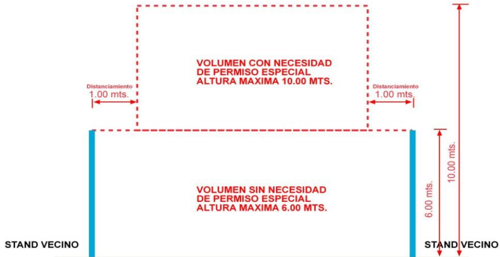
Esquema de elevación frontal
